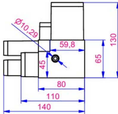
ÖN GÖRÜNÜŞÜ
