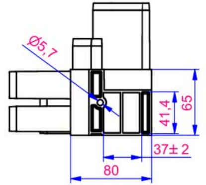
YAN GÖRÜNÜŞÜ
