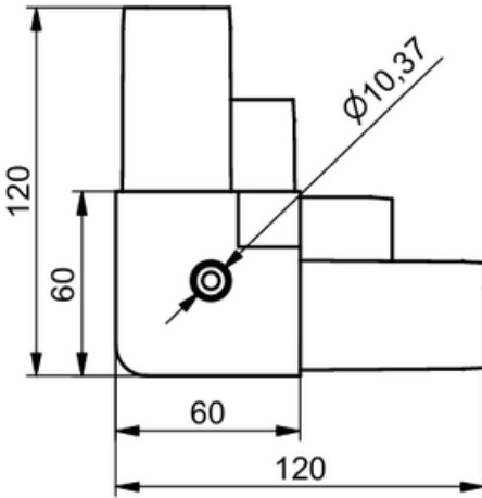
ÖN GÖRÜNÜŞ
