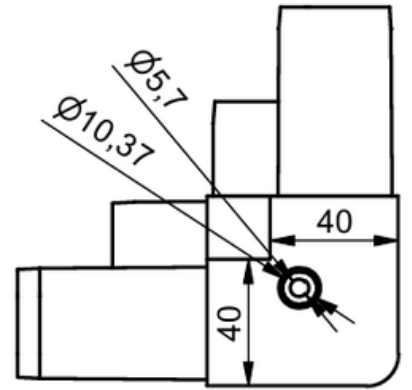
YAN GÖRÜNÜŞ
