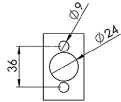
Dış ve İç Rozet Bağlantı Ölçüleri
