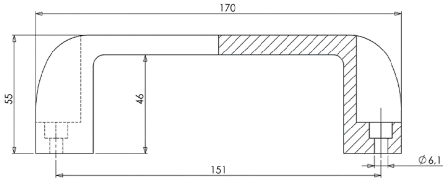
KESIT A-A
