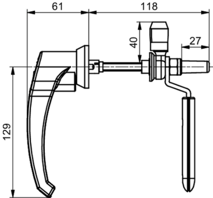
ÖN GÖRÜNÜŞ
