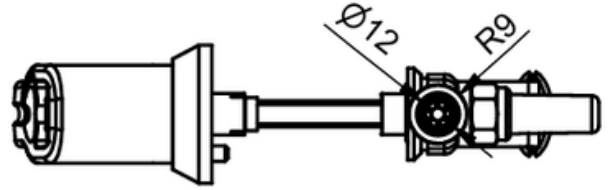
TABAN GÖRÜNÜŞ
