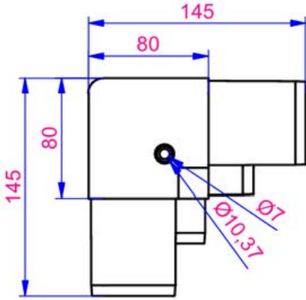
TABAN GÖRÜNÜŞÜ
