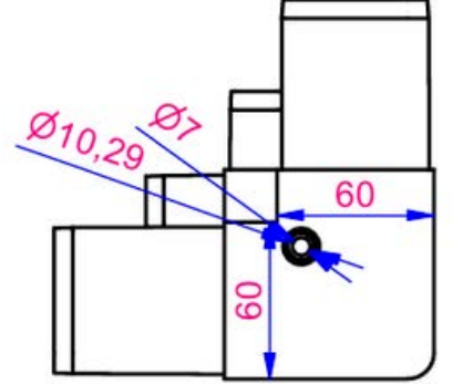
YAN GÖRÜNÜŞÜ
