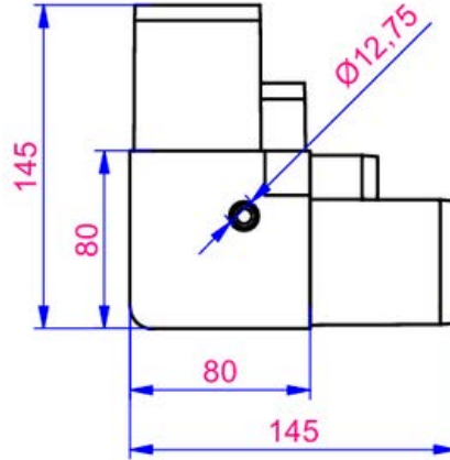
ÖN GÖRÜNÜŞÜ
