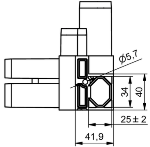
YAN GÖRÜNÜŞ
